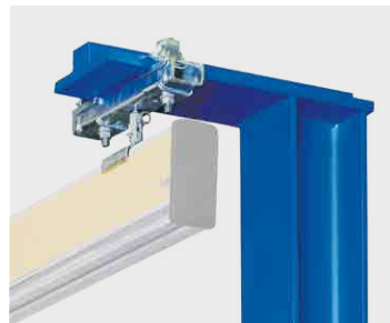
Kragarmstütze mit einseitiger Auskrantung
